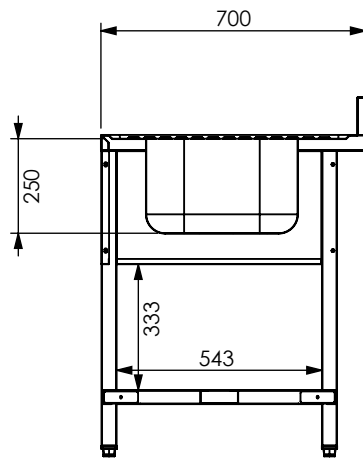
KESIT A-A
